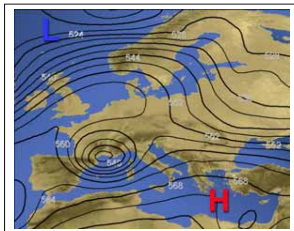
Campul de geopotential la 500 mb (ora 00)
