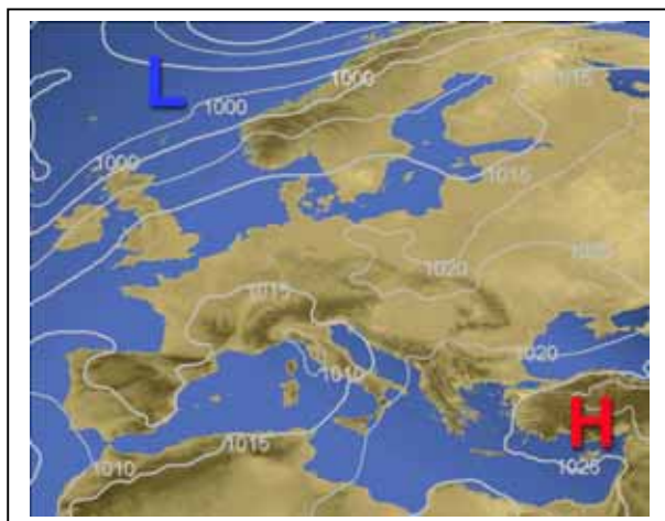
Presiunea atmosferica la nivelul mării (ora 00)
