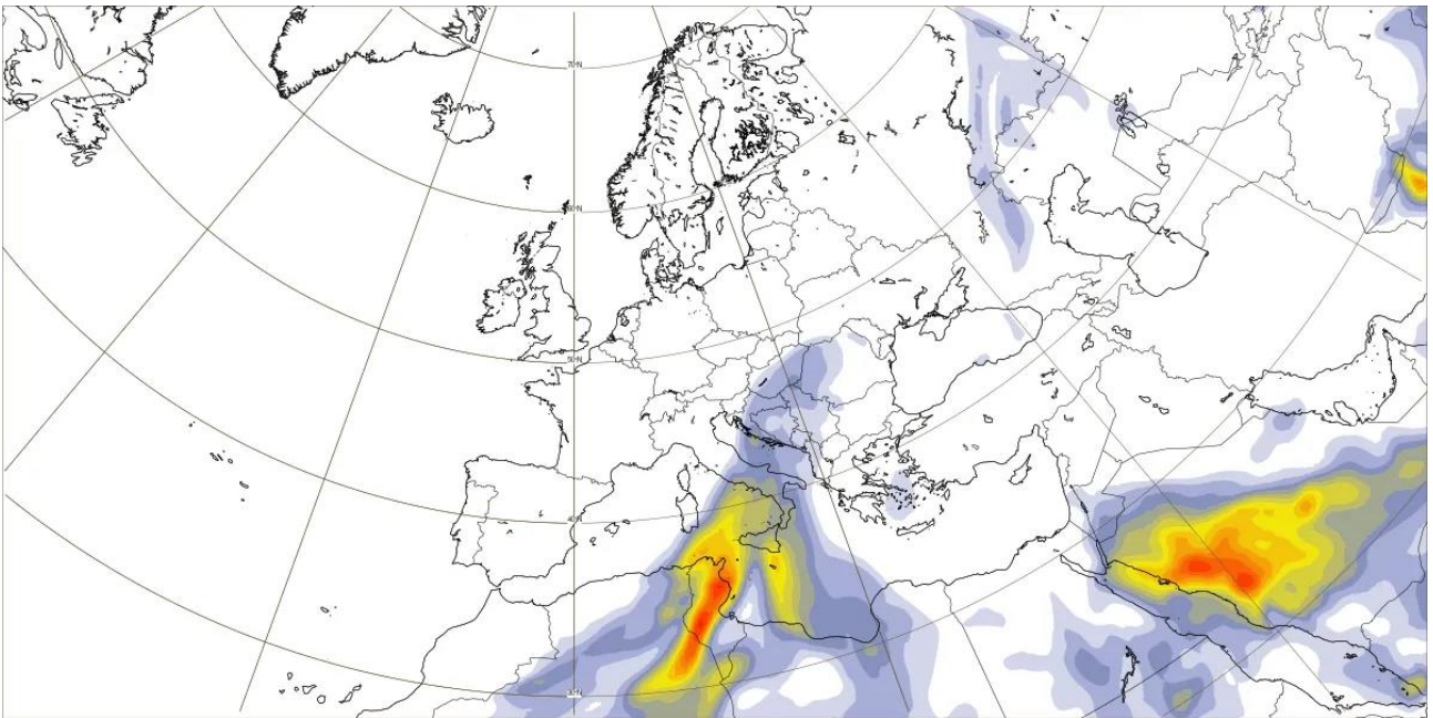
Evoluția masei de aer încărcate cu particule de praf 15 martie, ora 2
