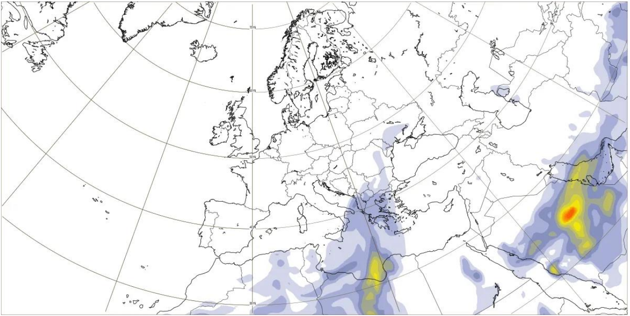
Evoluția masei de aer încărcate cu particule de praf 11 martie, ora 20
