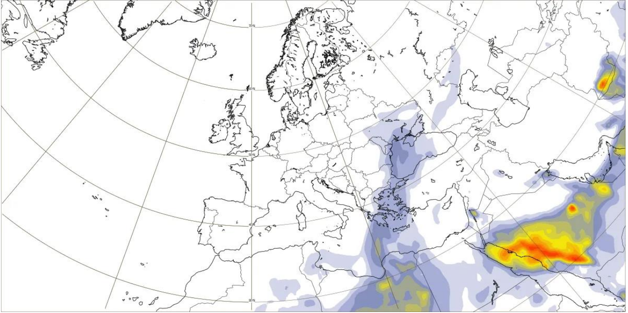
Evoluția masei de aer încărcate cu particule de praf 13 martie, ora 14
