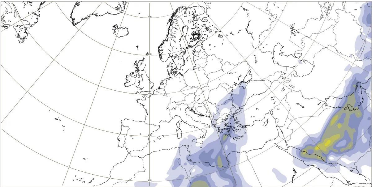
Evoluția masei de aer încărcate cu particule de praf 12 martie, ora 8
