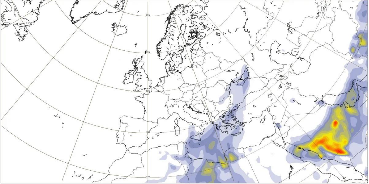
Evoluția masei de aer încărcate cu particule de praf 12 martie, ora 14
