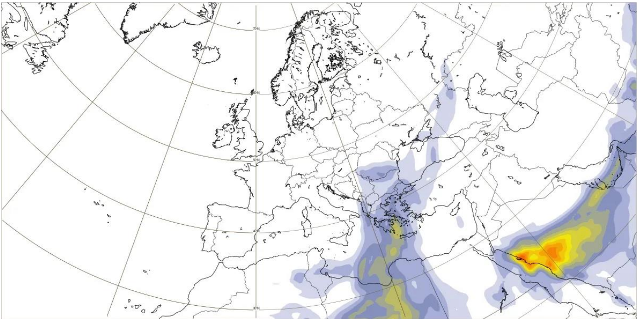
Evoluția masei de aer încărcate cu particule de praf 13 martie, ora 5
